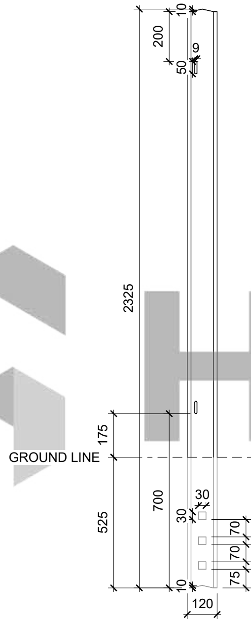
SCALE 1:15
